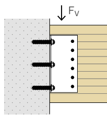
ALUMIDI med SBD självborrande dymlingar
