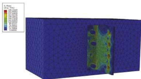
Solidmodell av ALU beslag på betong
